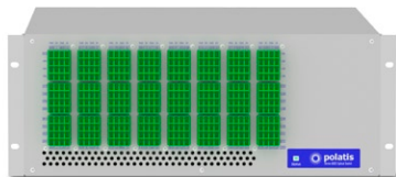
Polatis 192x192 Switch
